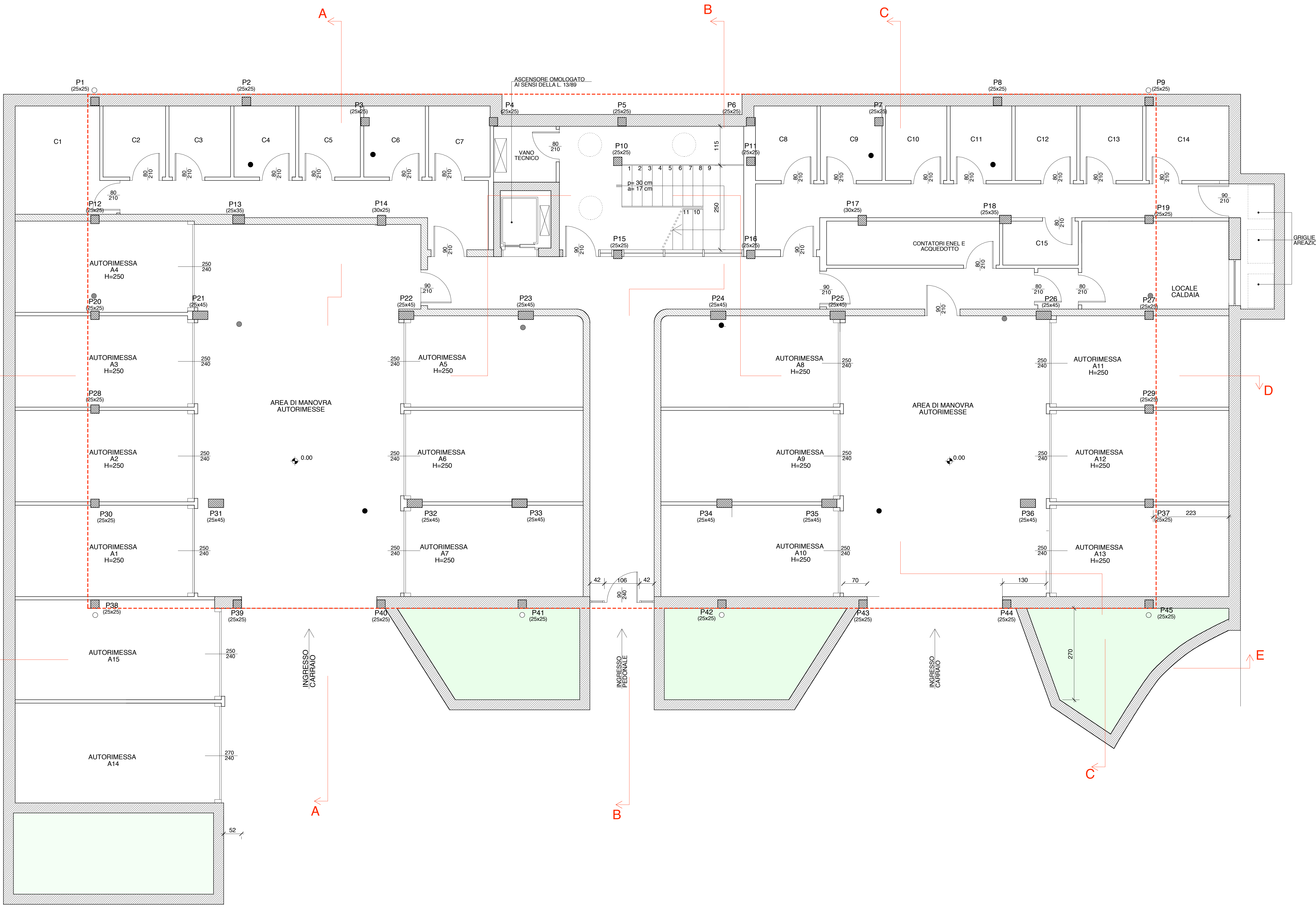
PIANTA PIANO TERRA SCALA 1/50
