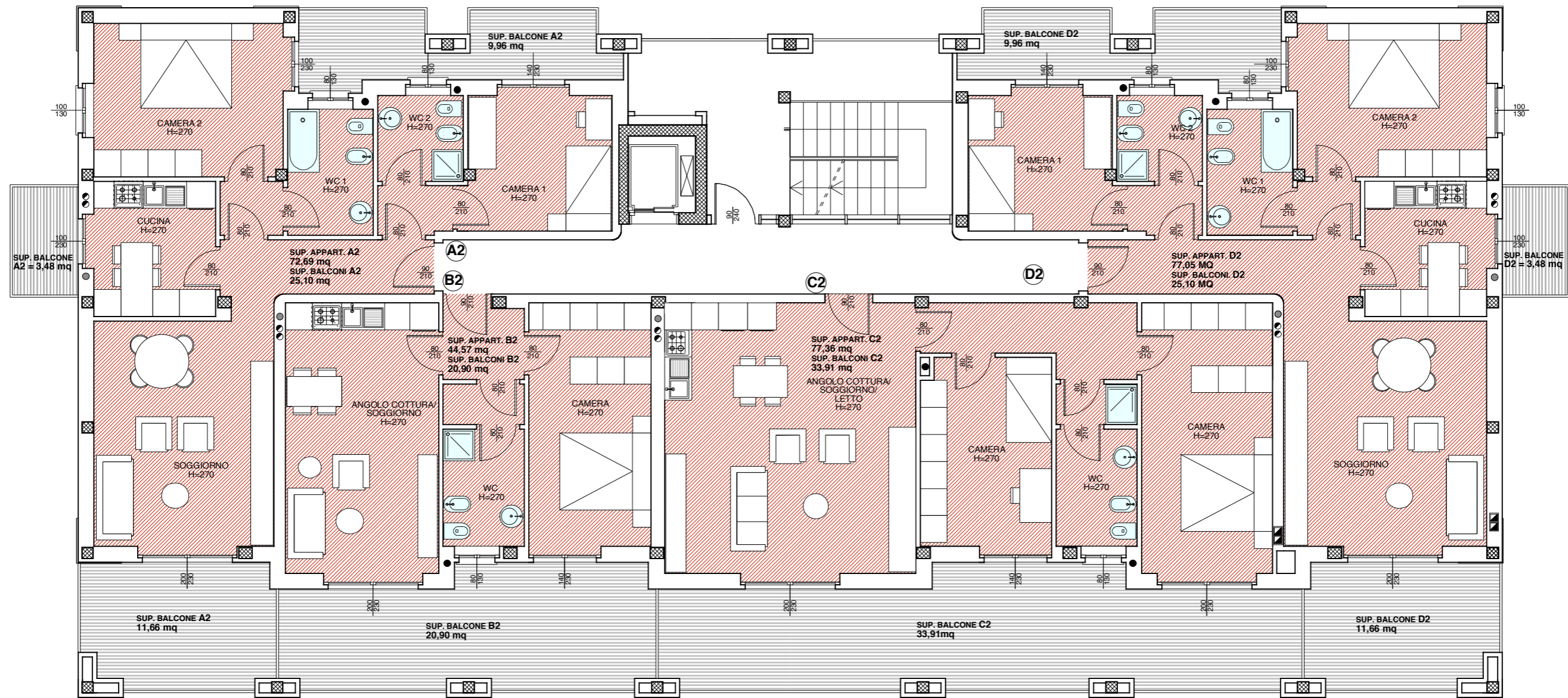
PIANTA PIANO SECONDO SCALA 1/100
